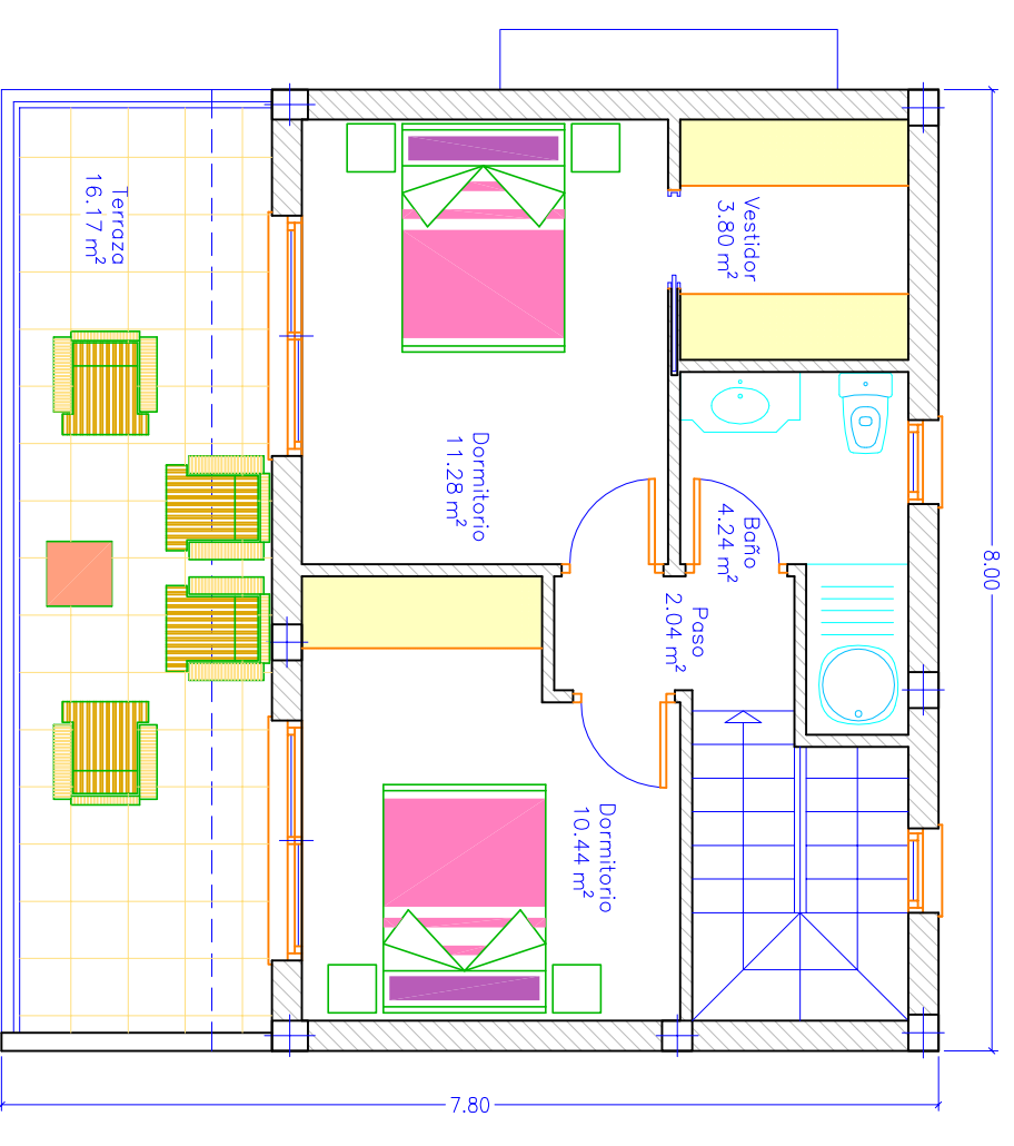
PLANTA ALTA Sup. construida=44,40m 2
